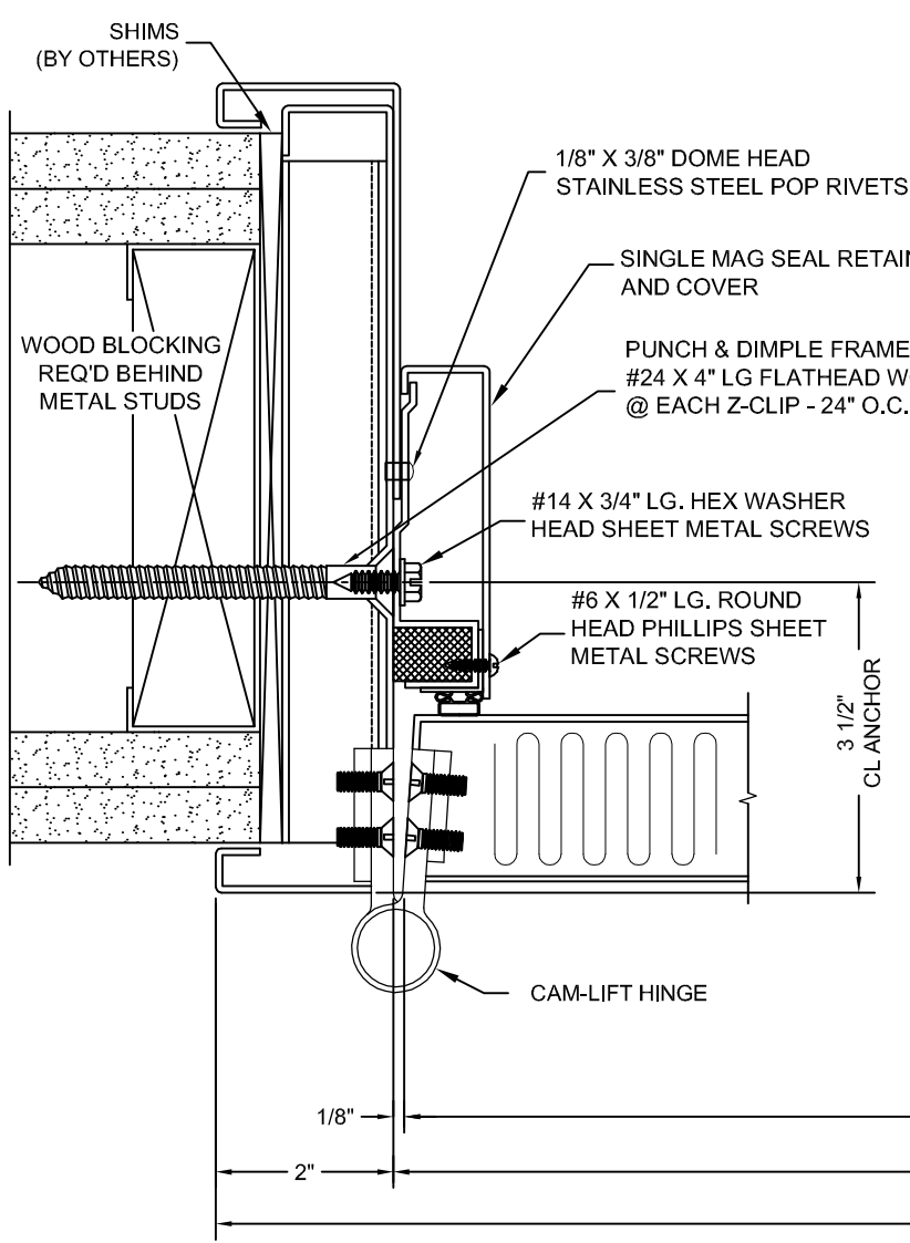
HINGE JAMB SECTION
